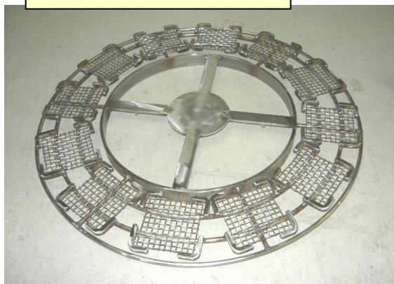
回転盤用ジグ
